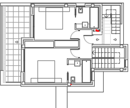
PLANTA PRIMERA ELEM. PRIV. Nº 1 TIPO D
