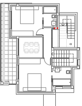
PLANTA PRIMERA ELEM. PRIV. Nº 2, 3, 4 y 5 TIPO A
